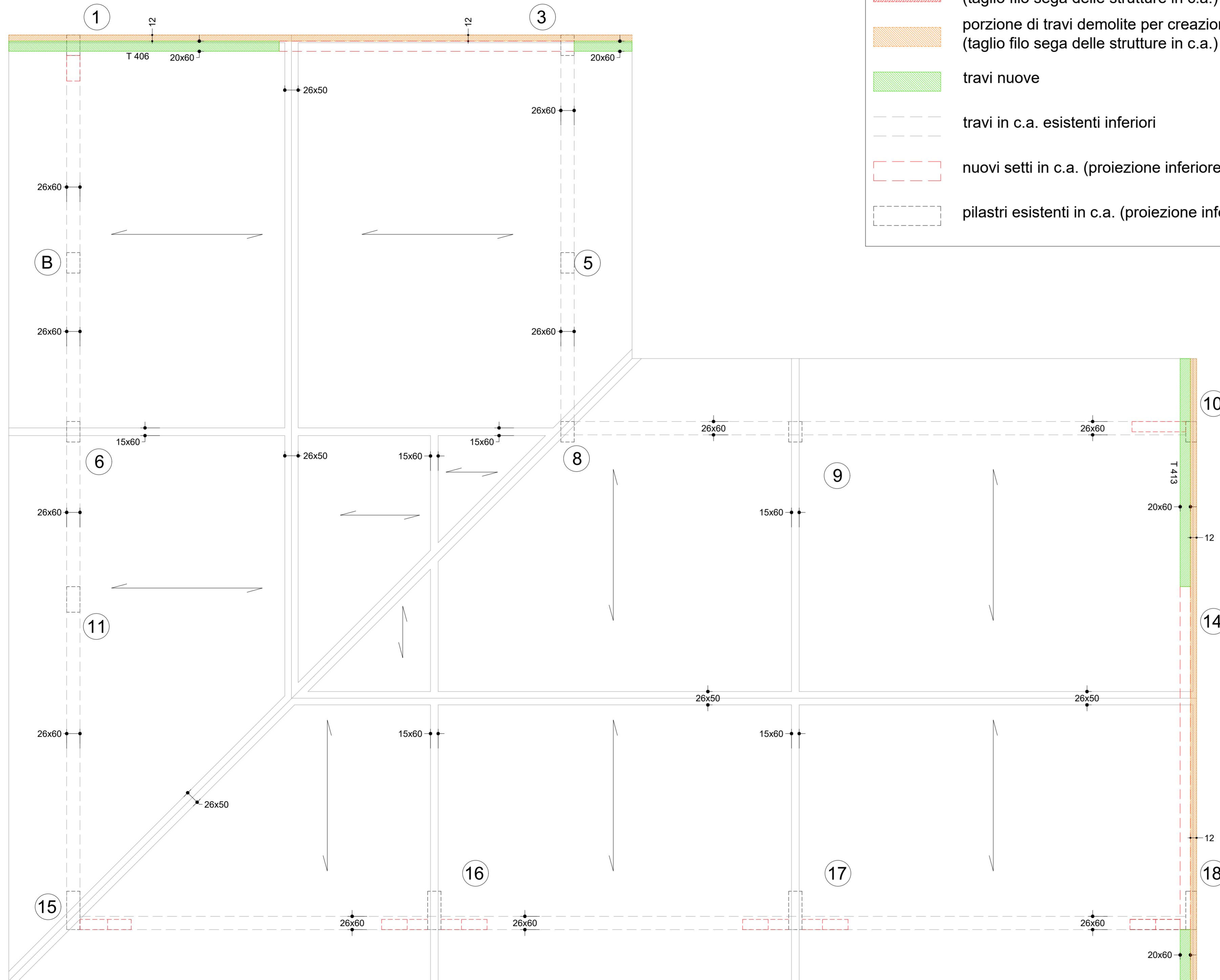
PIANO COPERTURA - STATO PROGETTO - SCALA 1:50
