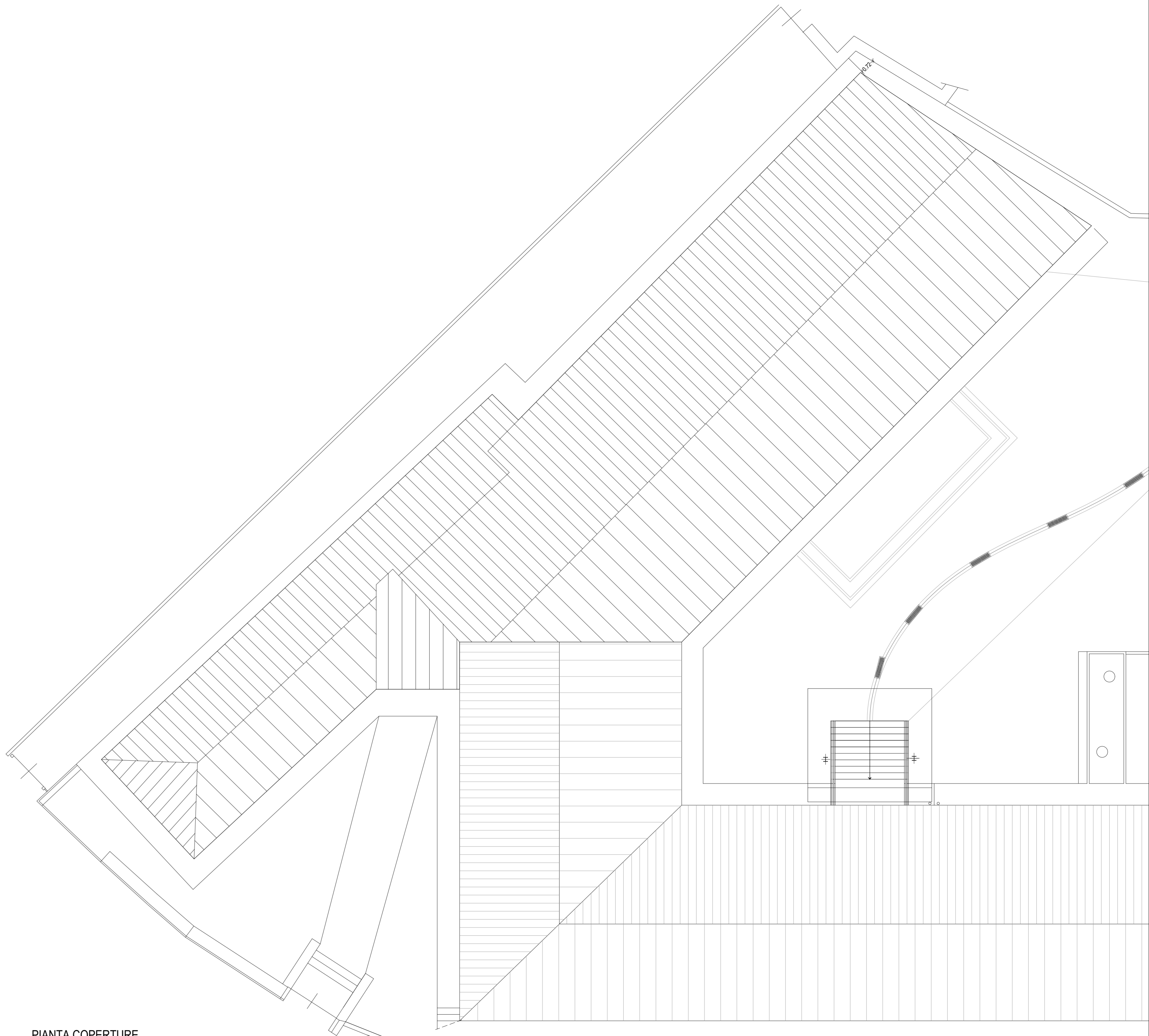
PIANTA COPERTURE
